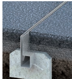
Typ ino 663 SR Schwerlastschlitzrinne befahrbar mit hohen Radlasten
