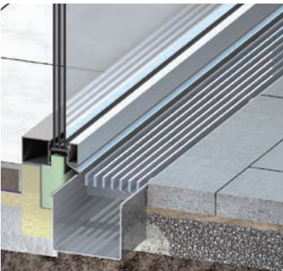
Typ ino 601 KR Standardrinne mit freier Rinneneinsicht für Fassaden
