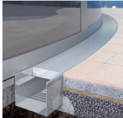
Typ ino 625 KR radiale Rinnenlösung mit durchgehender Rostauflage
