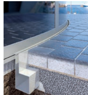
Typ ino 665 SR radial Radiale Schlitzrinne mit Schlitzweite 18 mm für den Einbau vor Fassaden
