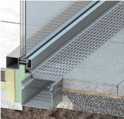
Typ ino 615 KR Standardrinne mit durchgehender Rostauflage und Einkantungen in den Aussenwänden
