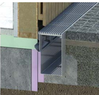
Typ ino 606 KR Rinne für den konstruktiven Holzschutz
